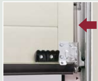
Kötélvezetés a kapulap és a tok között
